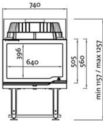
Jøtul I 570 πρόσοψη
