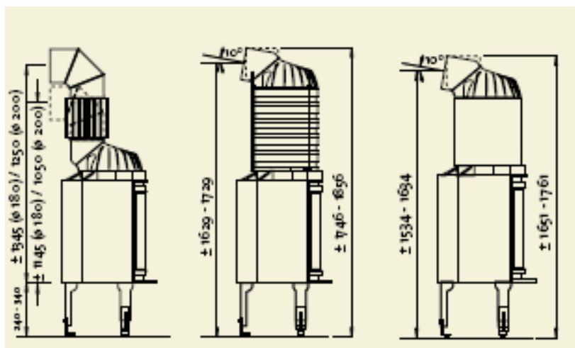
Jotul I18 Panorama πρόσοψη Jotul I18 Harmony πρόσοψη Jotul I18 τυπική σύνδεση
