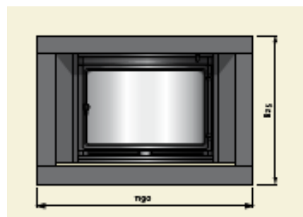
Ψηλό πλαίσιο για κάτω από το πέτρινο ράφι BP – μαύρη μπογιά
