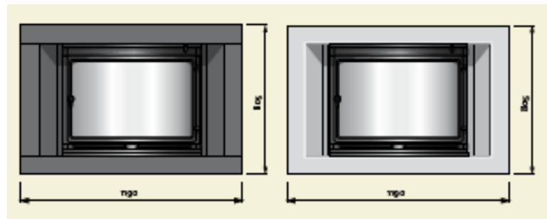
Ψηλό πλαίσιο BP – μαύρη μπογιά
