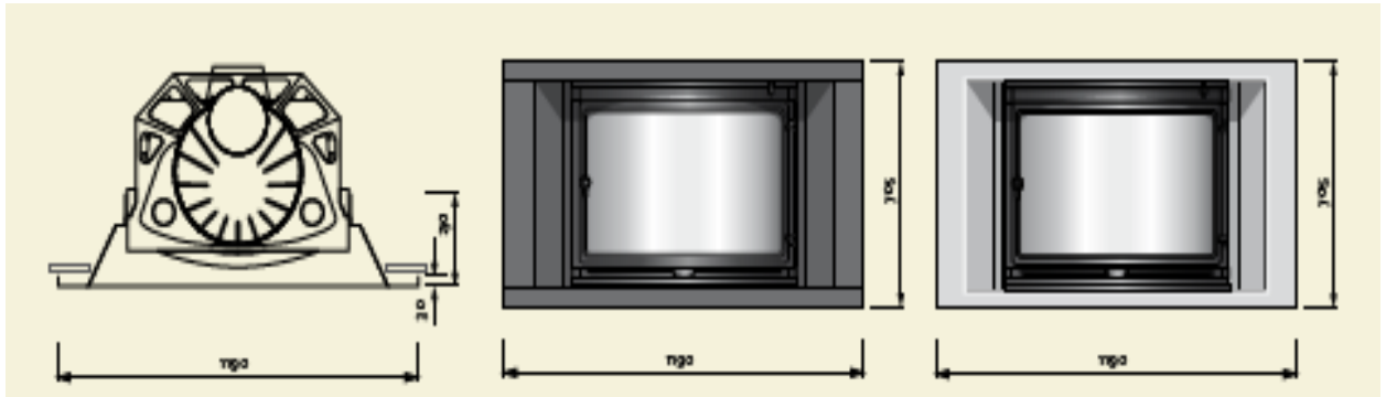
Ψηλό/κοντό πλαίσιο Jotul I18 ατσάλι από πάνω
