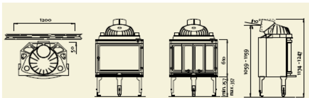
Jotul I18 Panorama πρόσοψη Jotul I18 Harmony πρόσοψη Jotul I18 τυπική σύνδεση
